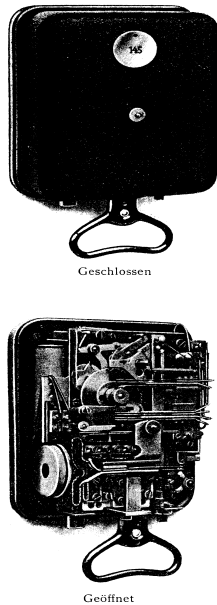
Abbildung 1: Polizei-Notruf-Privat-Hauptmelder
